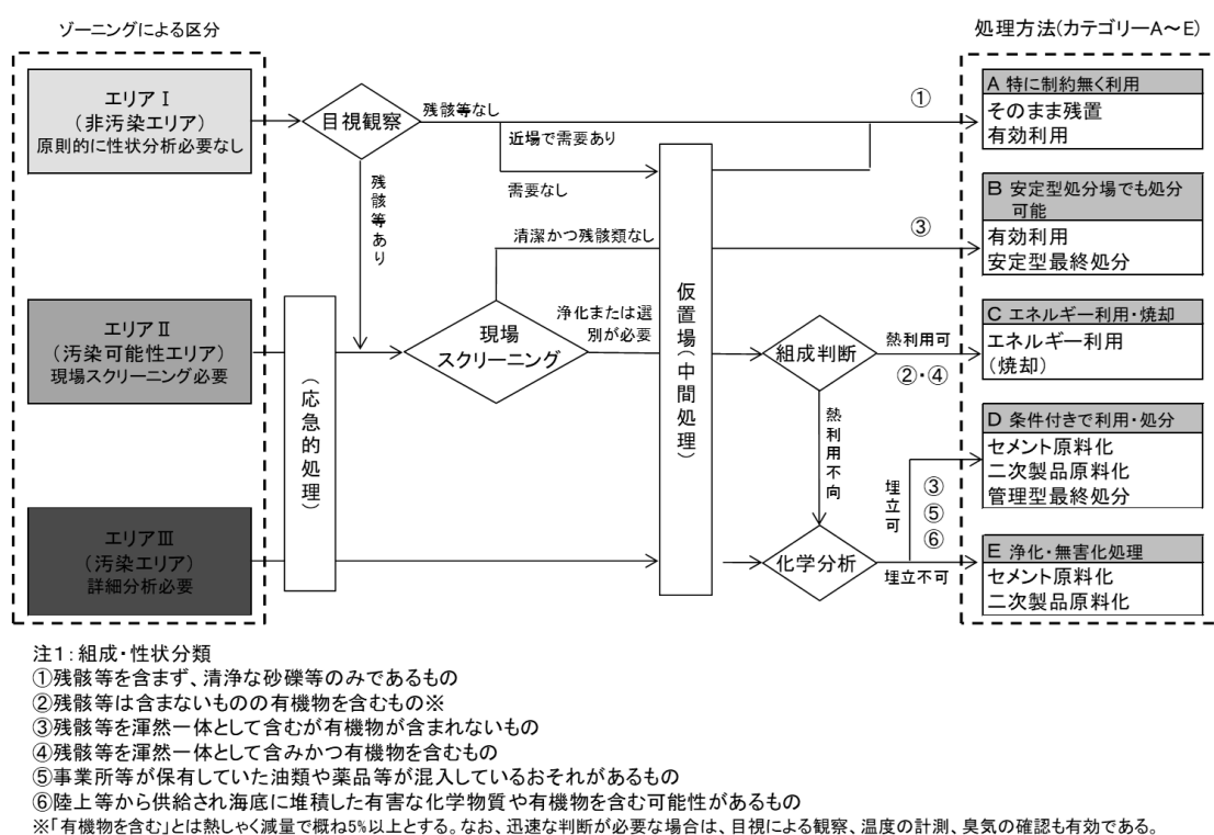
図15 津波堆積物の処理フロー
