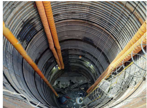
中間立坑埋戻し作業
