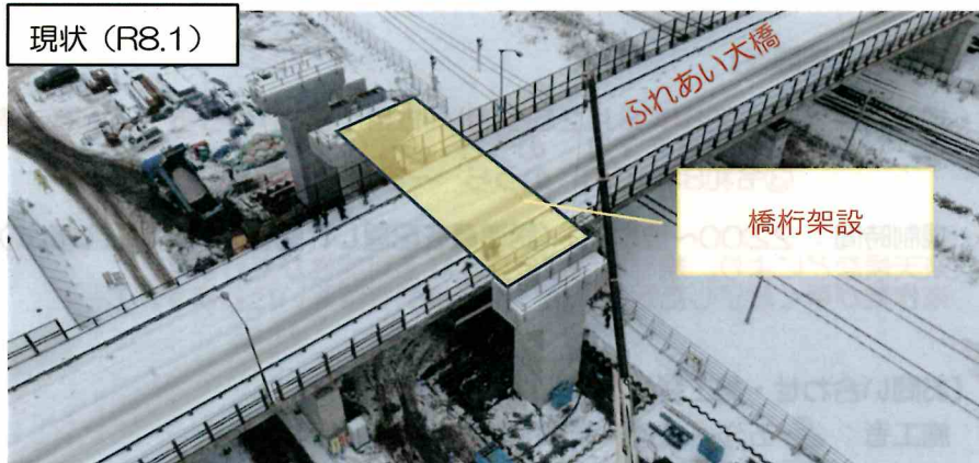
架設イメージ (2)
